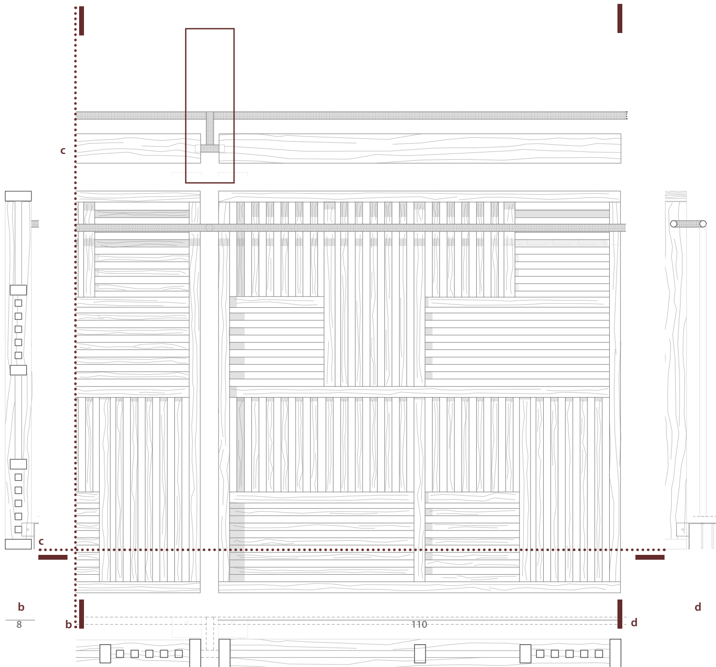
PARAPETTO e CORRIMANO
